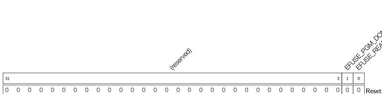
Register 20.27: EFUSE_INT_CLR_REG (0x114)
